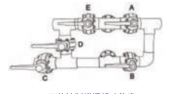
五位控制蝶阀组功能表 Five-position control butterfly valve group
