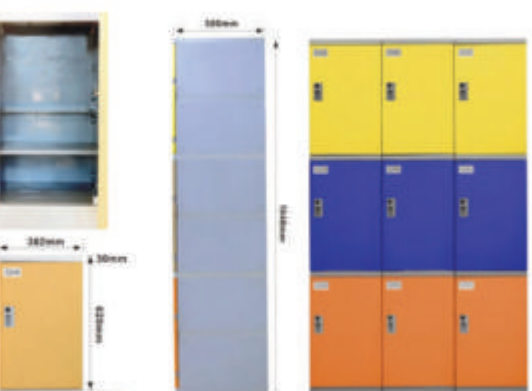
宽W 382 × 深D 500 × 高H 620mm
