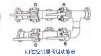
四位控制蝶阀组功能表 Four-position control butterfly valve group
